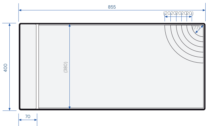
Bovenaanzicht
